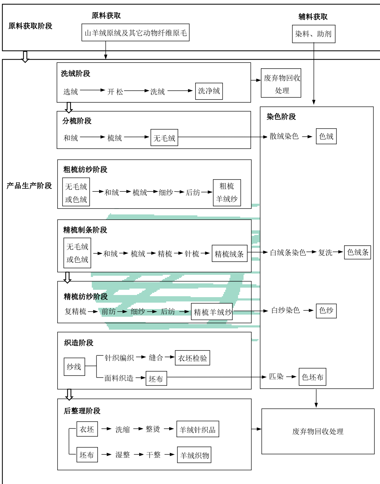
图 1 羊绒产品生命周期评价系统边界
